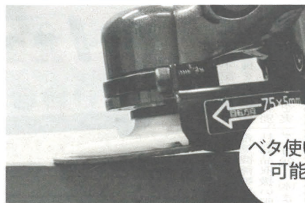
オフセット形状のため作業中に移動フランジが邪魔にならず、ベタ使いが可能
