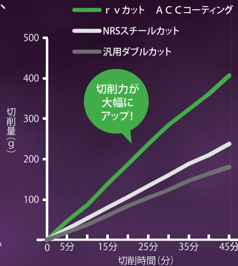
切削量比較
