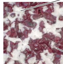
アルミ (A5052) 15分研削後面
