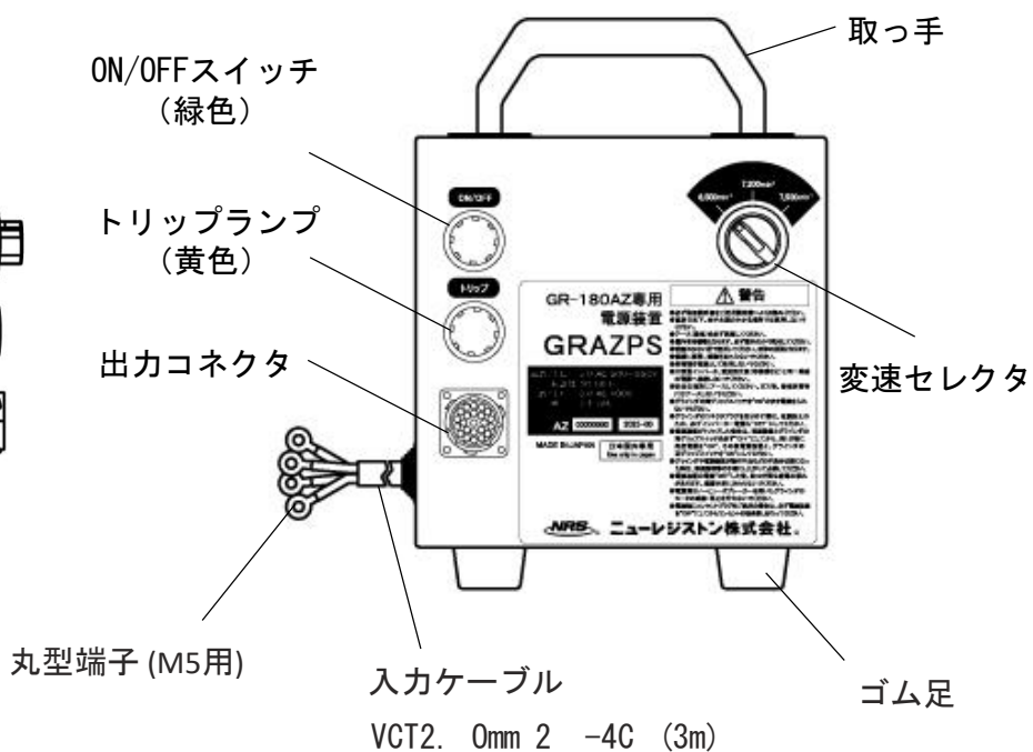
正面図
