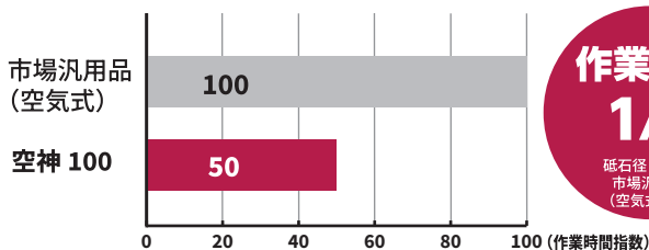
ブルーセラック外径 100mm #36 で 10 分間研削した場合の作業時間指数 (市場汎用品空気式グラインダを 100 とする)
